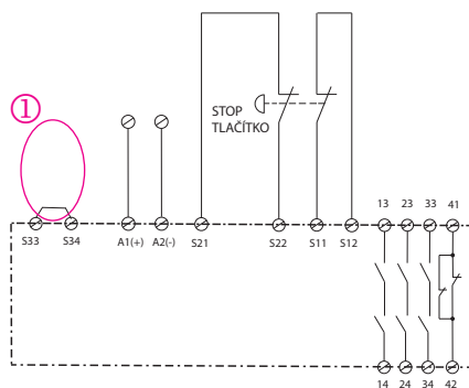
Dvoukanálový obvod nouzového vypnutí s opačnou polaritou mezi kanály
