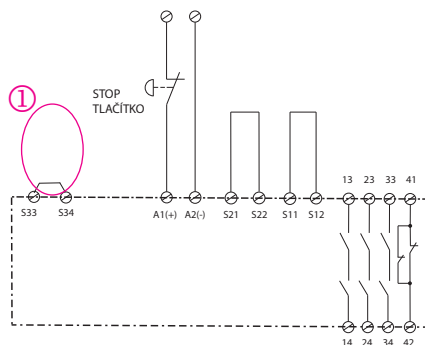
Jednokanálový obvod nouzového vypnutí
