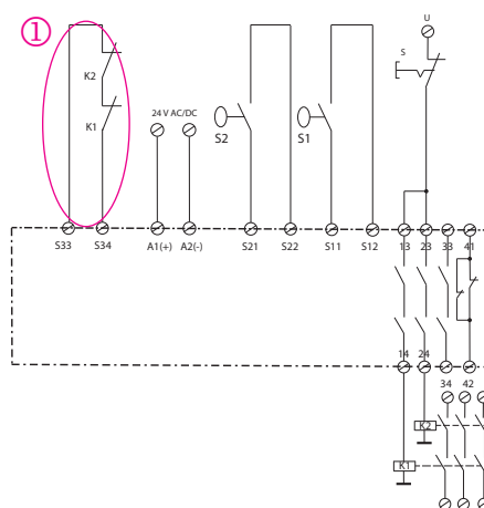
Dvoukanálové monitorování obvodu nouzového vypnutí s opačnou polaritou mezi kanály rozšířené o monitorování externích kontaktů
