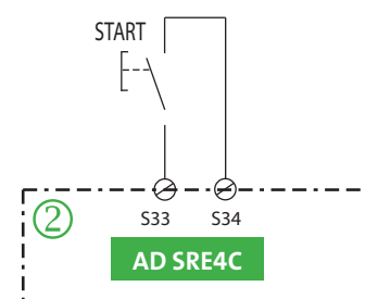
Manuální monitorovaný start/restart
