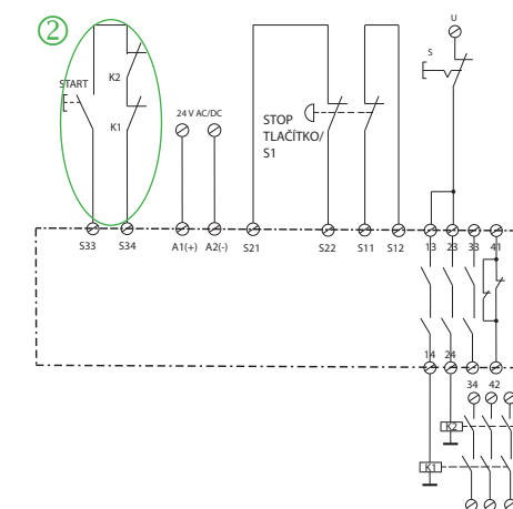
Dvoukanálové monitorování obvodu nouzového vypnutí s opačnou polaritou mezi kanály rozšířené o monitorování externích kontaktů
