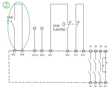
Dvoukanálový obvod nouzového vypnutí s opačnou polaritou mezi kanály
