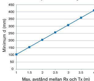
Monterings position (32 elements) Statisk och dynamisk montering
