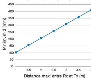
Position de montage (32 éléments) Montage statique et dynamique
