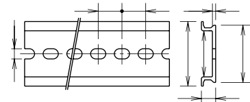
BAA/BAP
