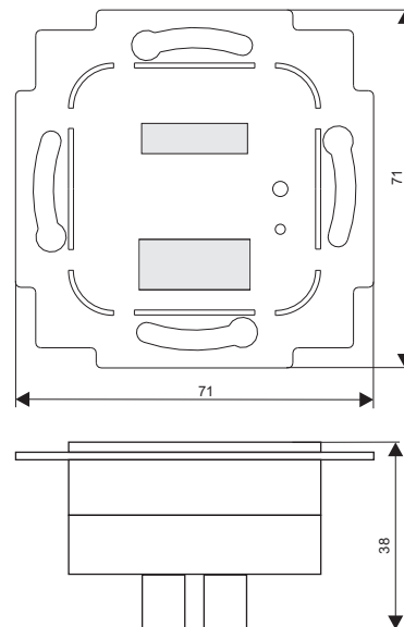
RS485-Schnittstelle RS485-Interface
