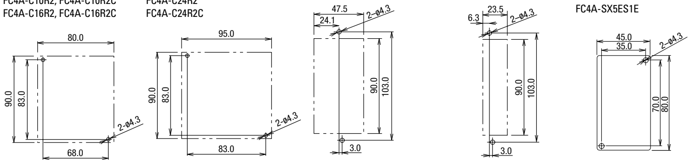
FC4A-SX5ES1E
