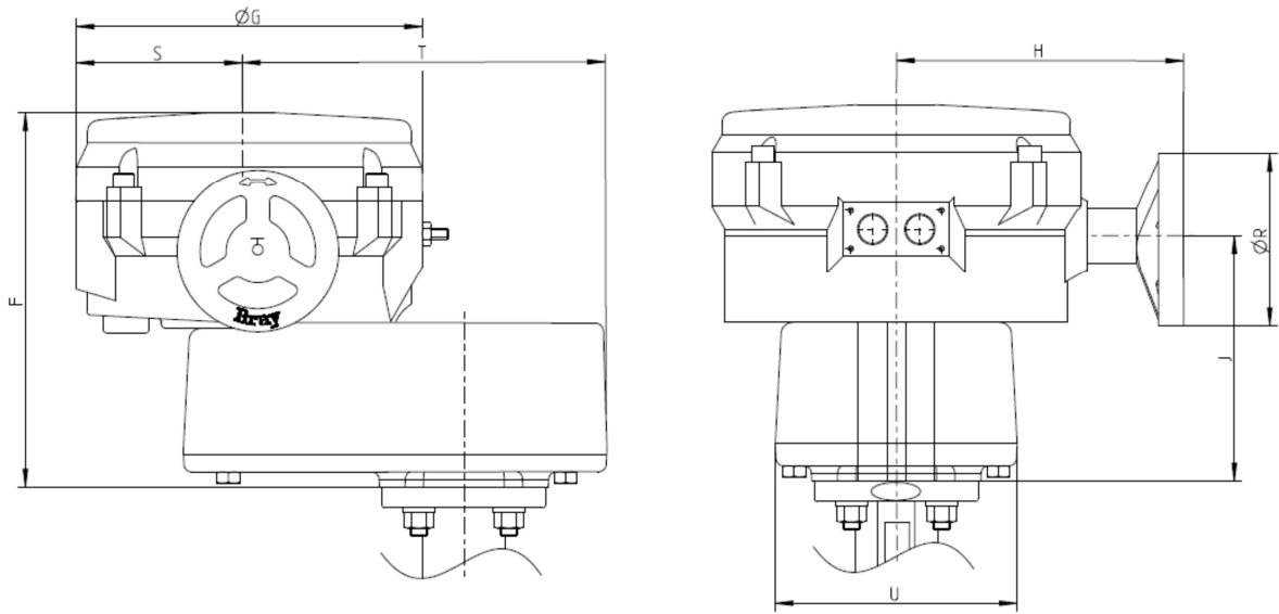
Fig. 7 S70M Actuator 130, 180
