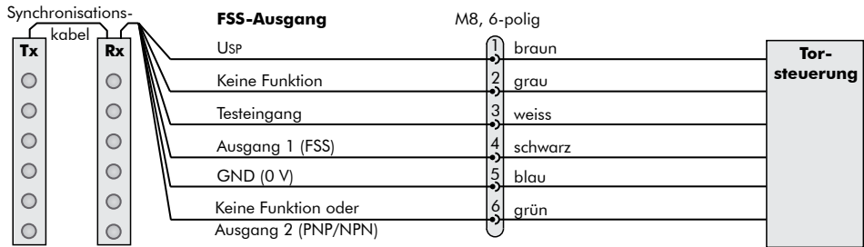
Abb 12: Anschlussdiagramm FSS-Ausgang
