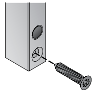
Abb 10: Frontale Montage
