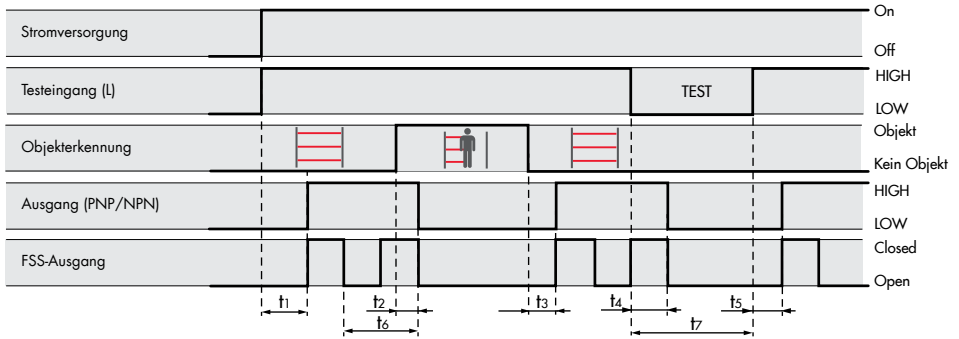
Abb 14: Zeitdiagramm
