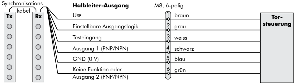
Abb 11: Anschlussdiagramm Halbleiter-Ausgang
