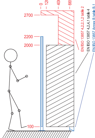
Bezpečnostní vzdálenost ve výšce 2200 mm
