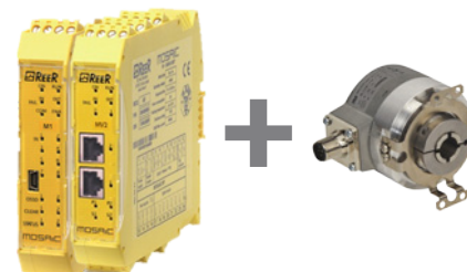
bezpečnostní jednotka MOSAIC + jeden SAFECODER = SIL 3
