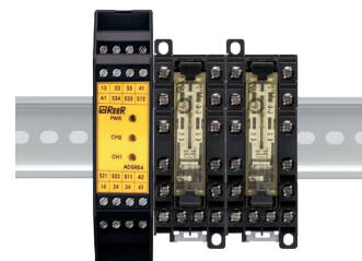
Příklad ekonomického rozšíření výstupů bezpečnostního relé
