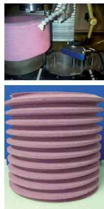
Měření a kontrola profilu brusných kotoučů
