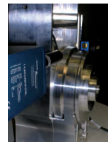
Kontrola excentricity hnacího kotouče
