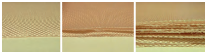
Stanovení počtu vrstev tkanin při výrobě airbagových polštářů
