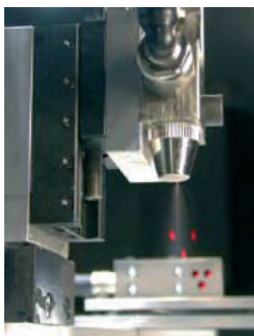
Kontrola kvality postříku – detekce ucpaných nebo špatně nastavených trysek
