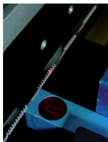
Kontrola symetrického umístění žhavicího vlákna žárovky
