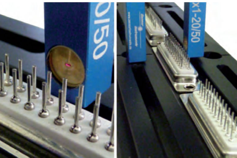
Kontrola výšky a šířky pinů u elektronických součástek
