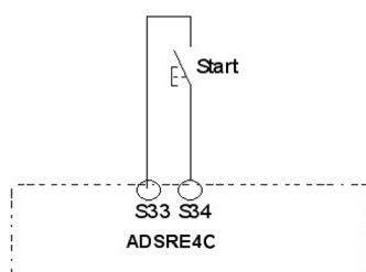
Manuální monitorovaný start/restart
