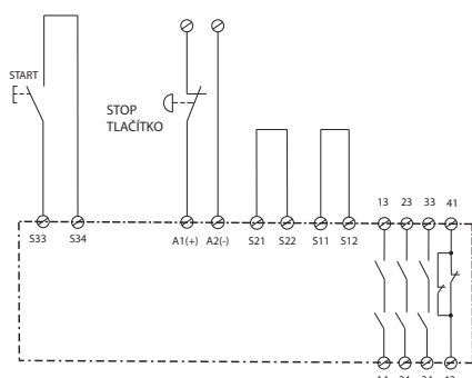
Jednokanálový obvod nouzového vypnutí
