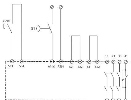
Monitorování bezpečnostní brány
