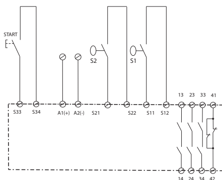
Dvoukanálové monitorování bezpečnostní brány s opačnou polaritou mezi kanály
