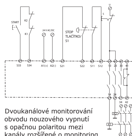
Dvoukanálový obvod nouzového vypnutí s opačnou polaritou mezi kanály
