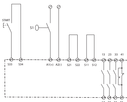
Monitorování bezpečnostní brány
